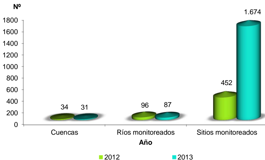
Gráfica 4-3. CUENCAS, RÍOS Y SITIOS MONITOREADOS: AÑOS 2012-2013
